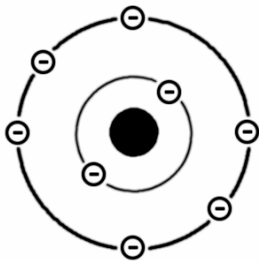
Átomo de oxígeno incluyendo sus 8 electrones
