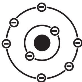
Sauerstoff-Atom inkl. seiner 8 Elektronen
